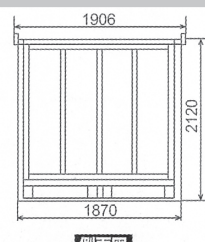
側面図
