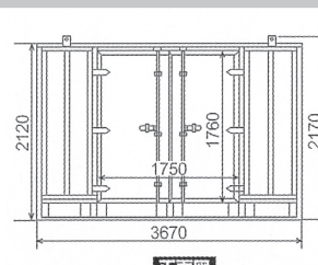
正面図
