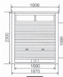
正面図
